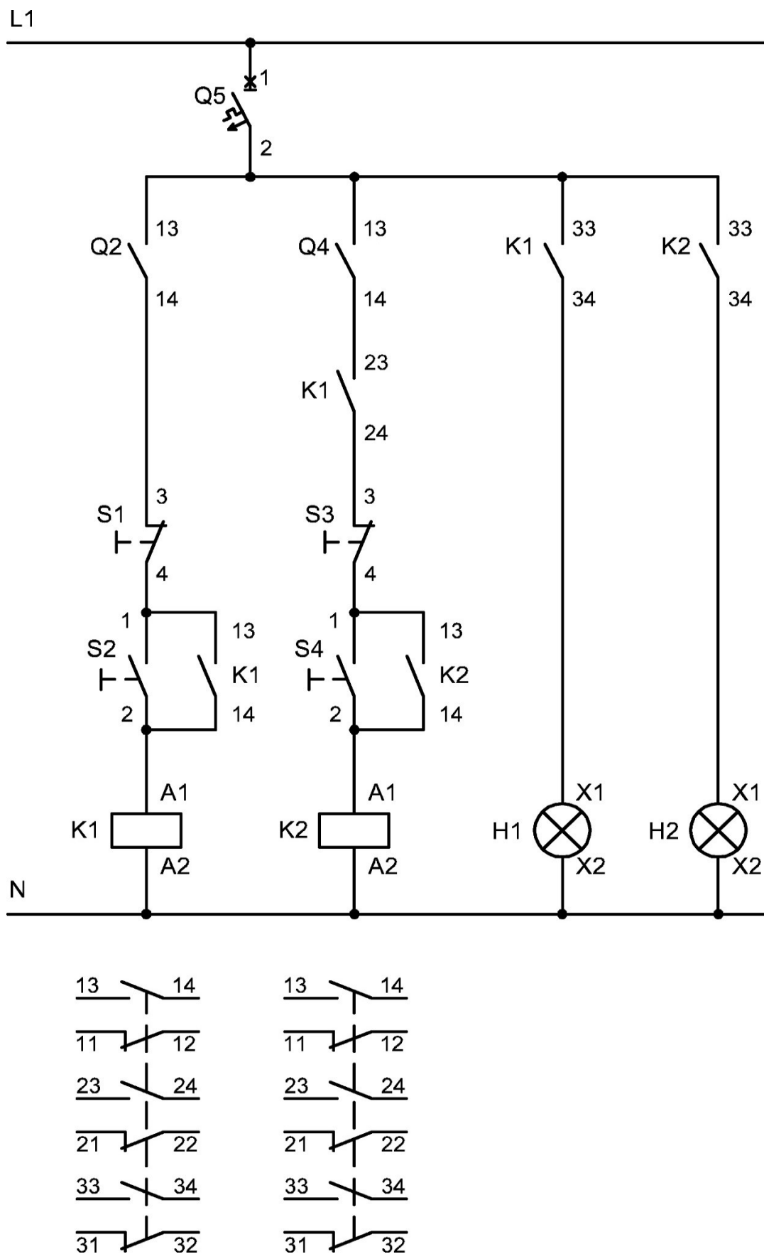
Rysunek 2. Schemat obwodu sterowania układem pracy dwóch silników
