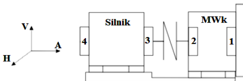
Schemat z punktami pomiarowymi na obudowach łożysk
