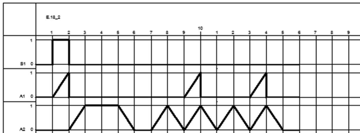
Rys. 3. Diagram czasowy
