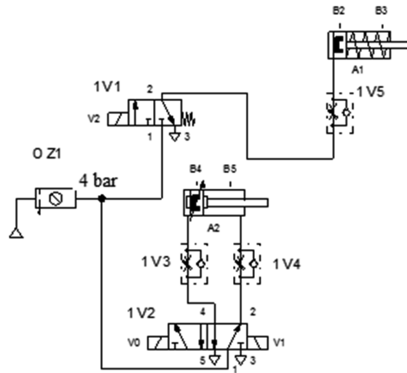
Rys. 2. Schemat połączeń pneumatycznych
