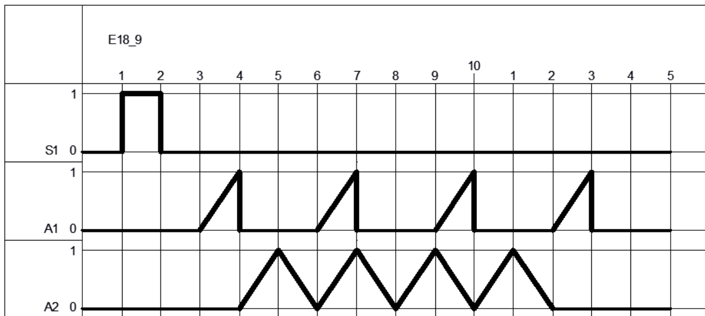
Rys. 4. Diagram czasowy. Wymagana dokładność trwania poszczególnych faz \pm 0,5 s
