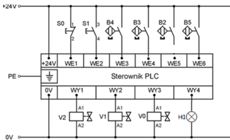
Rys. 2. Schemat podłączenia elementów elektrycznych do sterownika PLC.
