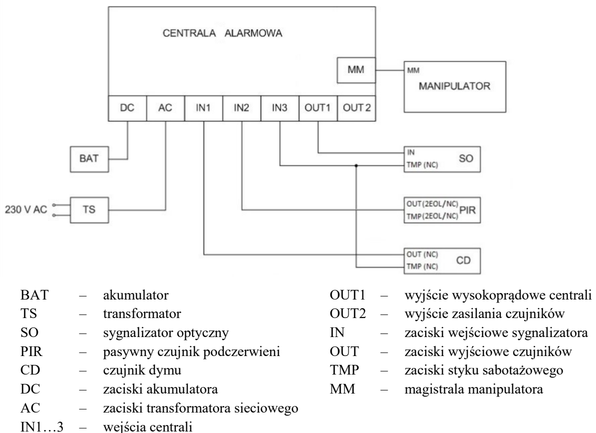
Rysunek 1. Schemat montażowy instalacji alarmowej
