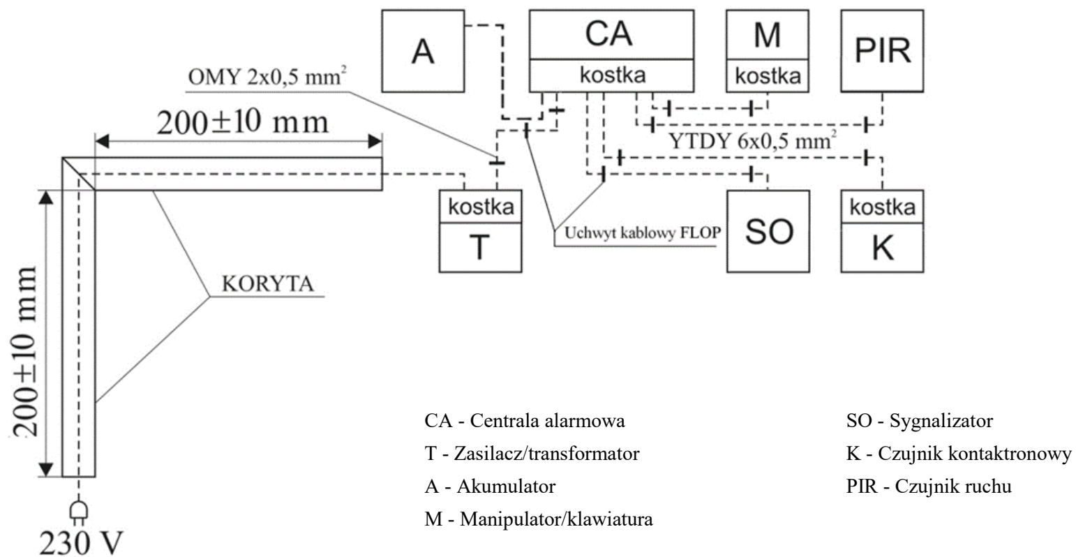
Rys. 1. Schemat połączeń instalacji alarmowej
