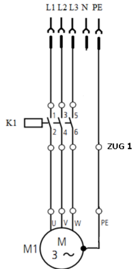
Rysunek 4. Schemat połączeń zasilania silnika trójfazowego
