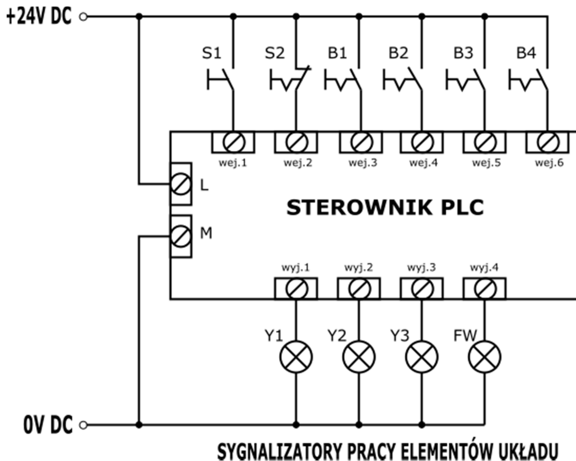
Rysunek 1. Schemat połączeń układu do testowania programu sterowniczego.
