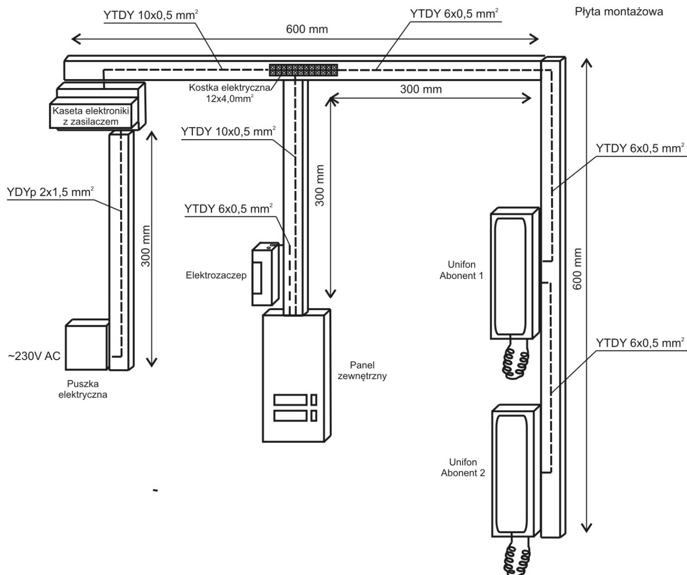
Rysunek 1. Schemat rozmieszczenia elementów instalacji domofonowej.
