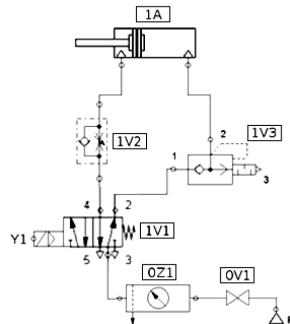
Rys. 2. Schemat połączeń pneumatycznych układu elektropneumatycznego
